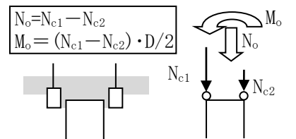
図3 Aにおける釣合い
